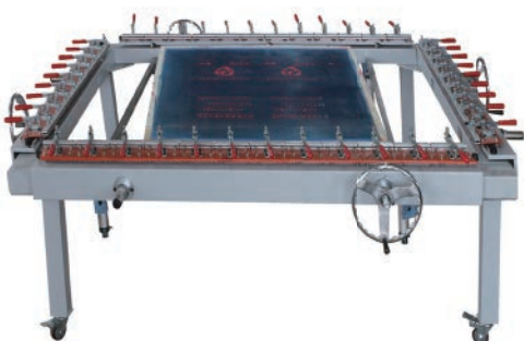
气动拉网机 Pneumatic Net Machine
