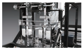
Double Ultrasonic Sealing 双道超声波封口
